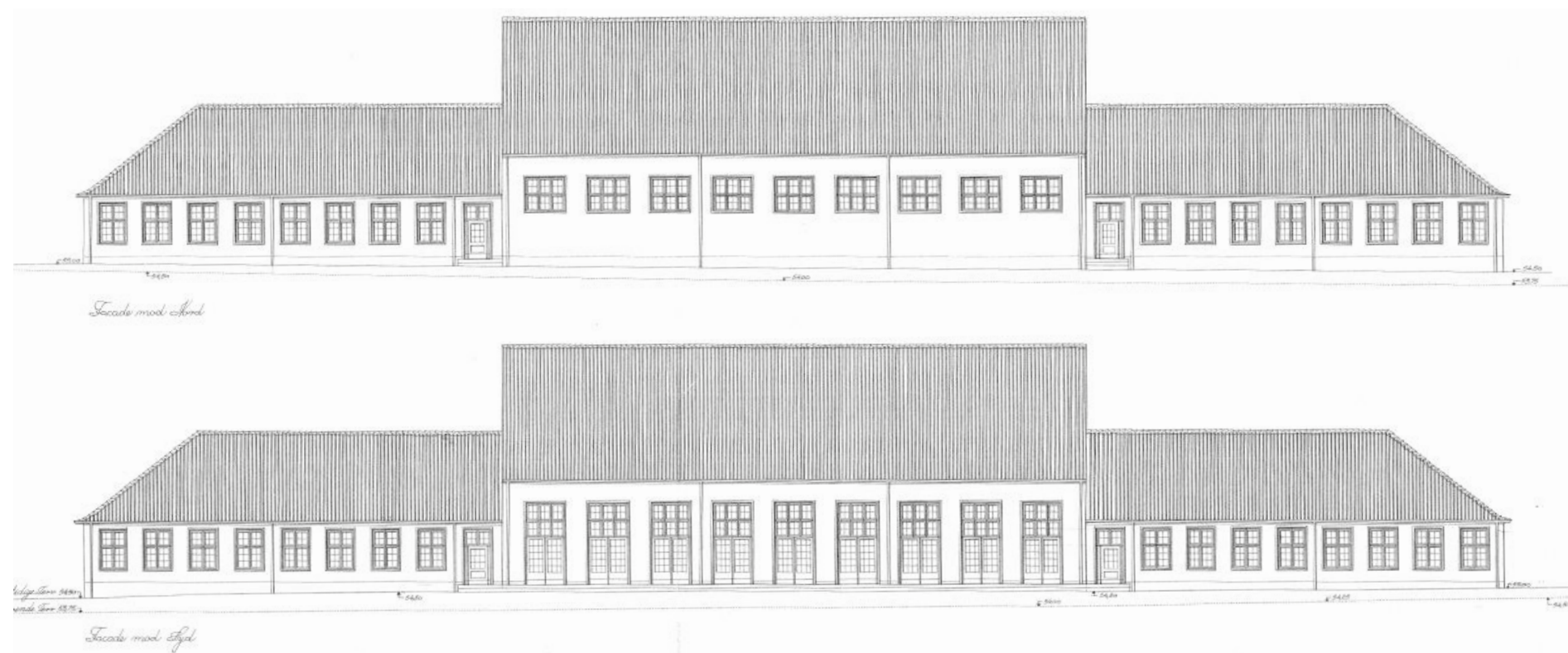
Eksisterende facader - syd og nord
