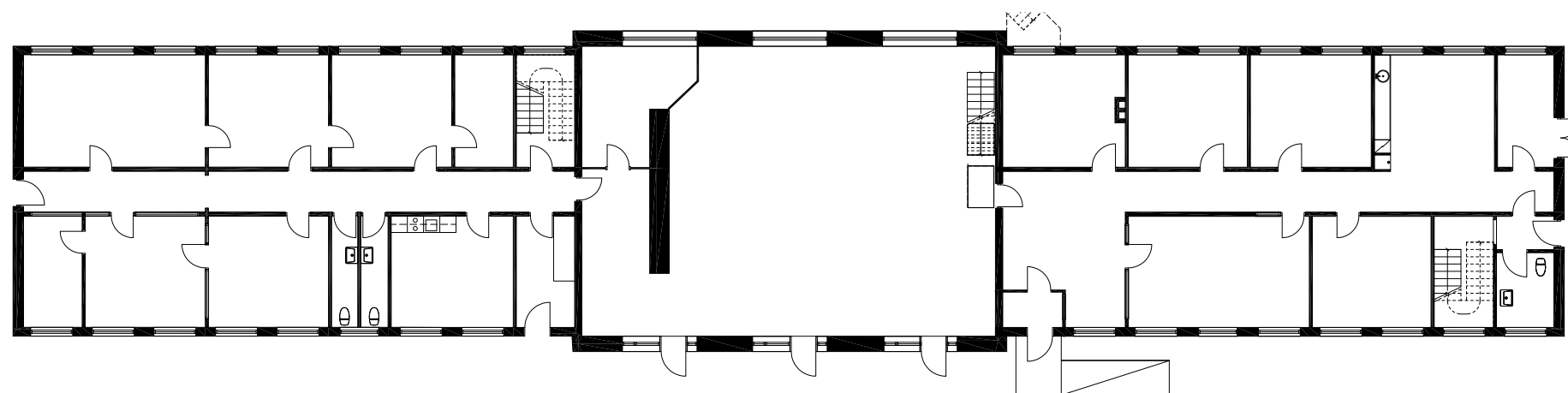
Eksisterende stueplan
