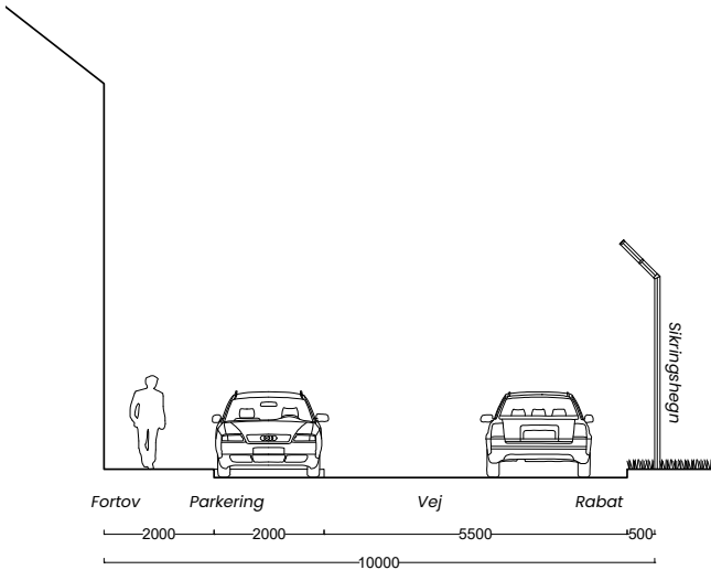
Principsnit AA for vejudlæg indenfor sikringshegn
